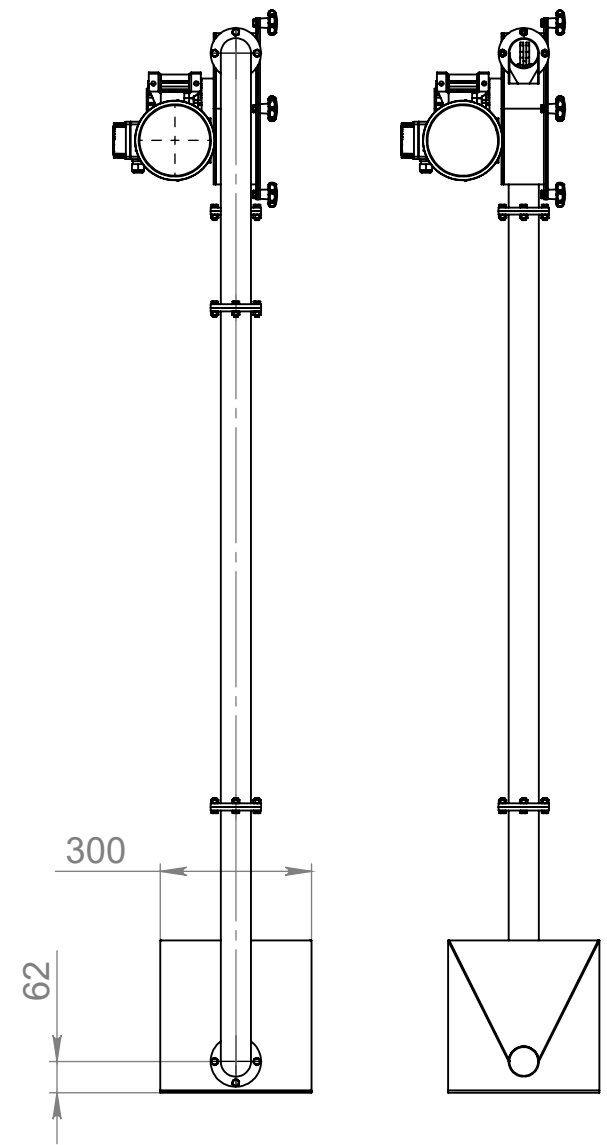
A-A (1 : 15)
